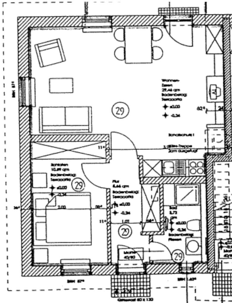
Grundriss
